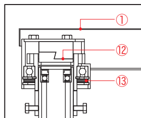
①完成羽根内部拡大図
