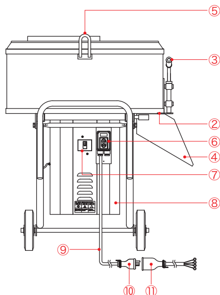
■100V仕様部分図
