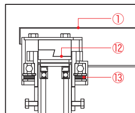
①完成羽根内部拡大図
