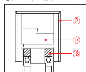
②完成羽根内部拡大図
