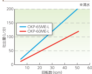
回転数－吐出量特性表
