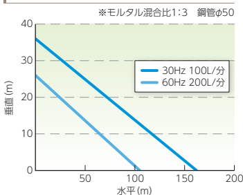
輸送距離(水平－垂直)特性表 OKP-65ME-L
