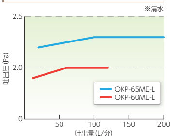
吐出量－吐出圧特性表
