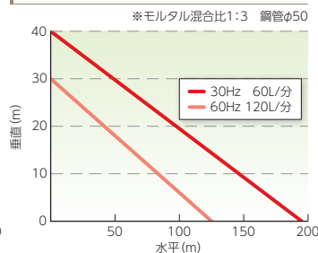
輸送距離(水平－垂直)特性表 OKP-60ME-L
