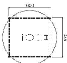
■750φプラスチックホッパー寸法図
